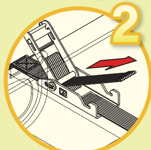
フック取付・ベルト緊張 (※足場板側面と平行になるよう、フックを押付けてください。)
